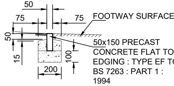
EDGING TYPE E1 SCALE 1:20
