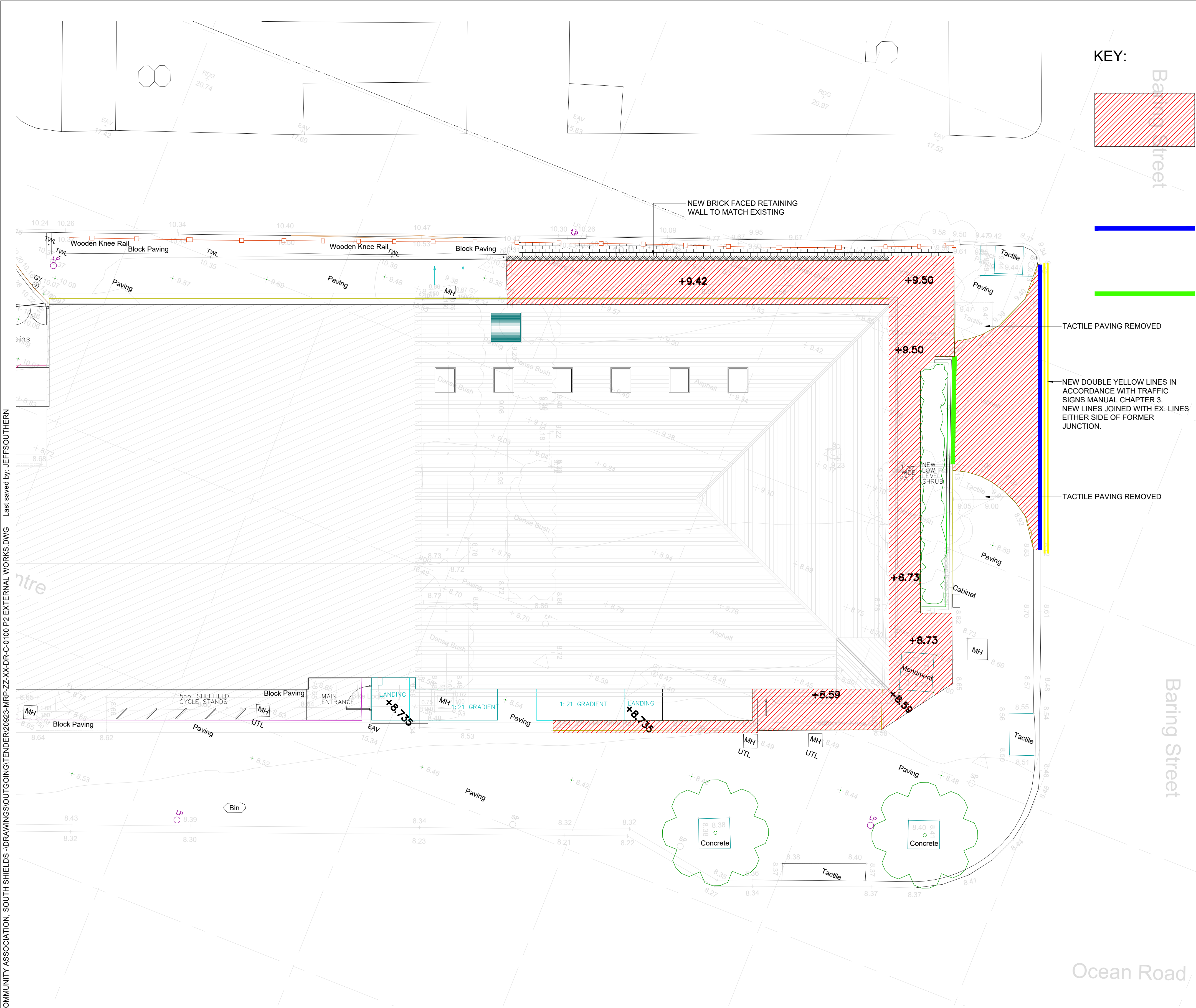
1 SITE LAYOUT 1:100
